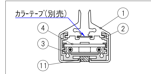
A-A 断面図 (1/1)
